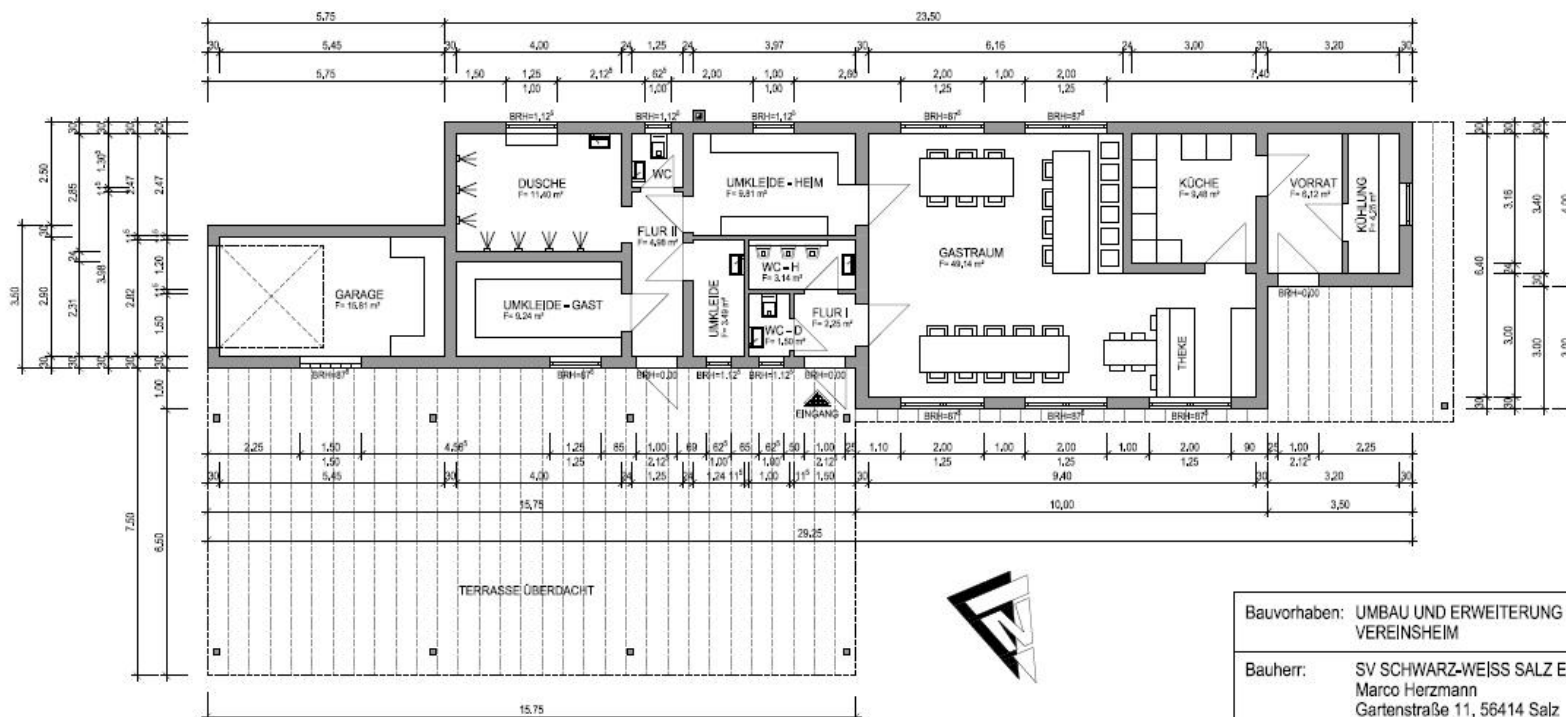
BESTANDSPLAN
